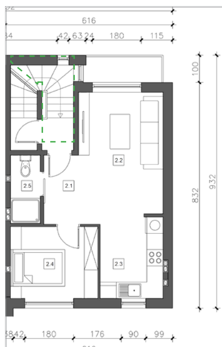
PIĘTRO I
