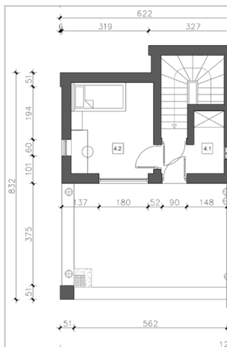
PODDASZE
