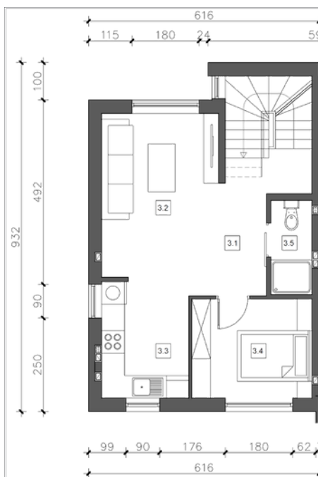
PIĘTRO II
